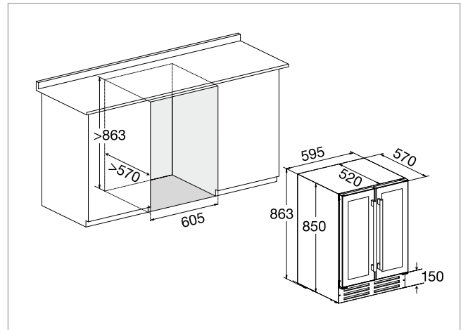
Model: WP2DQ60DCS, WP2DQ60DCB
