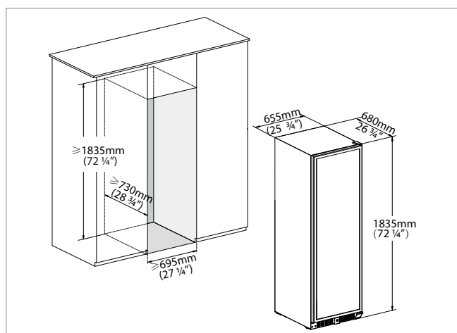
Model: E1000DRB, E1000DRW, E1000DX, CPR01800SRB, CPR01800SX
