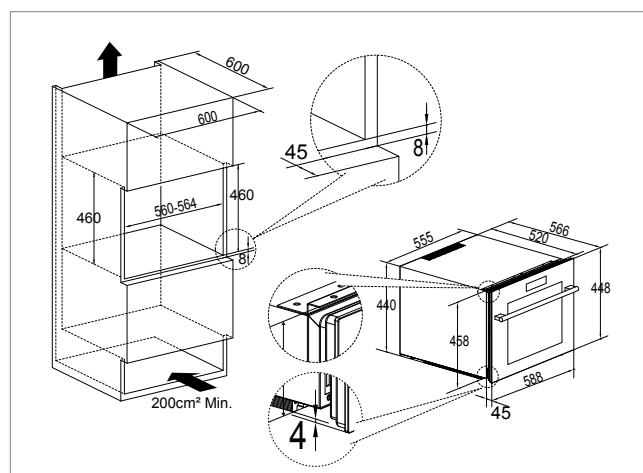
Model: OZ45SBTOP, SOMZ45SB
