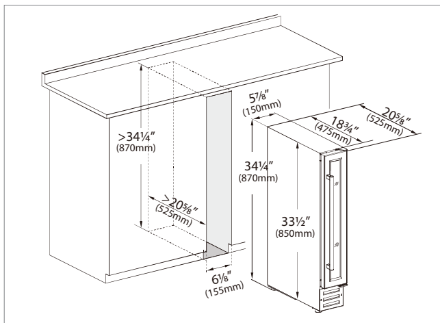
Model: WPQ15SCS, WPQ15SCB
